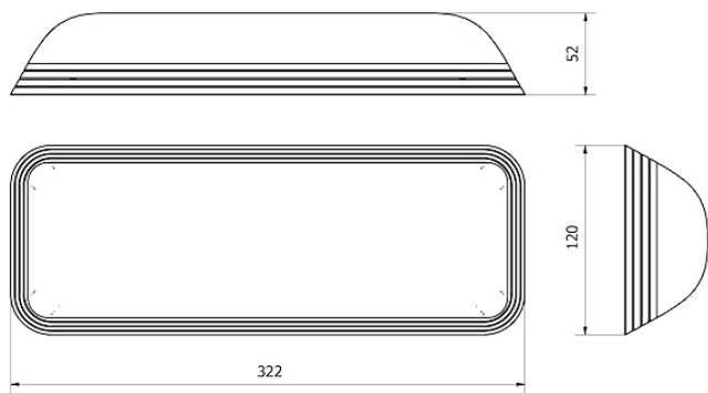
Dimensiones (mm):
