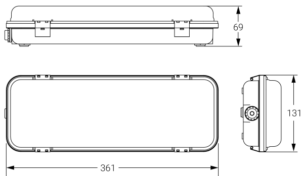
Dimensiones (mm):
