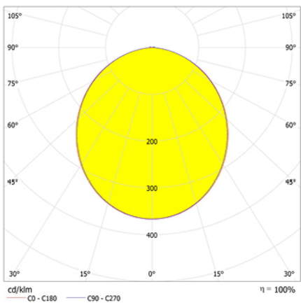
Datos fotométricos:
