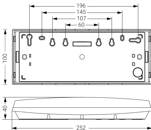
Dimensiones (mm):
