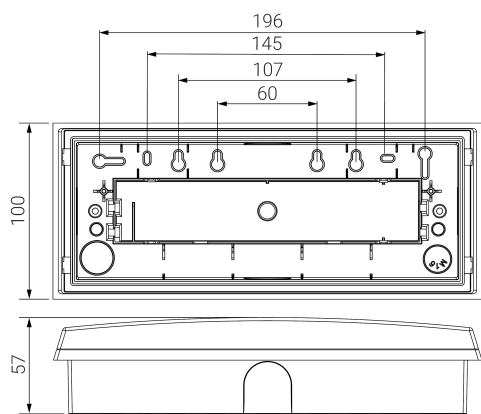
Dimensiones (mm):
