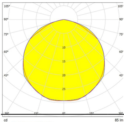
Datos fotométricos:
