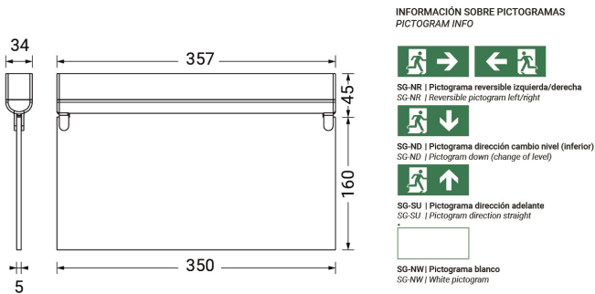
Dimensiones (mm):
