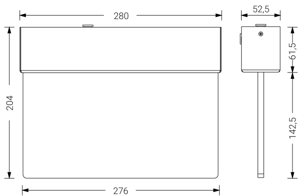
Dimensiones (mm):
