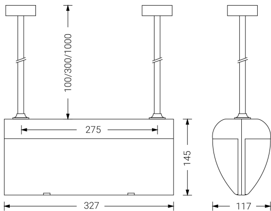
Dimensiones (mm):
