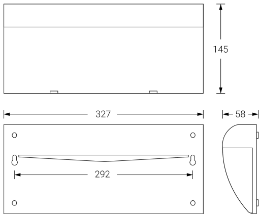
Dimensiones (mm):
