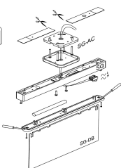
Montaje fijación a techo Ceiling fixation
