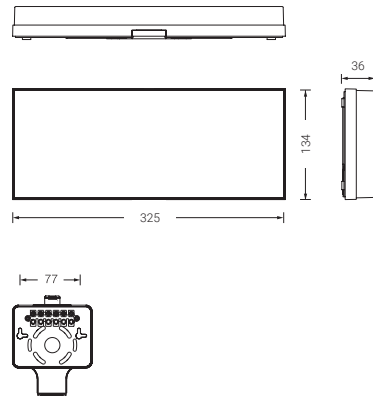
Base enchufable
